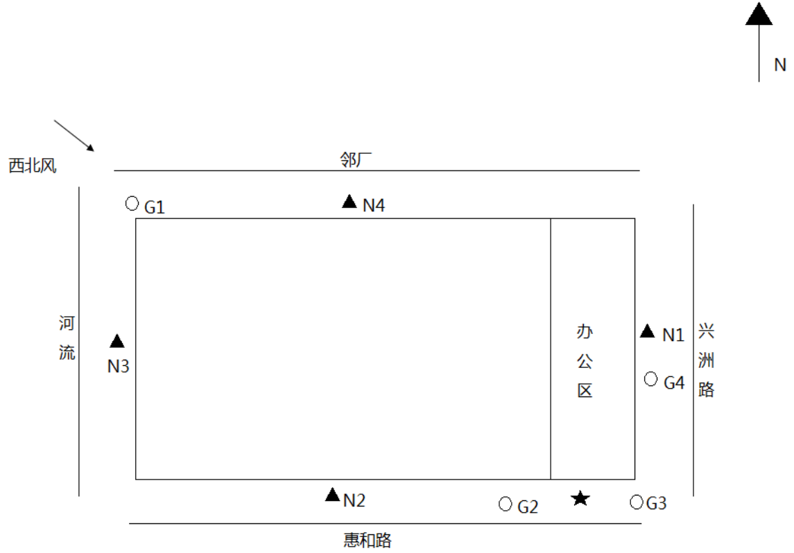
图 3-3 验收监测点位示意图（监测 2 天点位一致）
