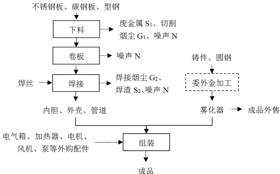
图 2-2 本项目生产工艺流程及产污环节图
